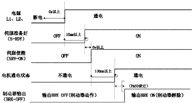
图 5-4 电源接通时接收伺服开启信号的时序
