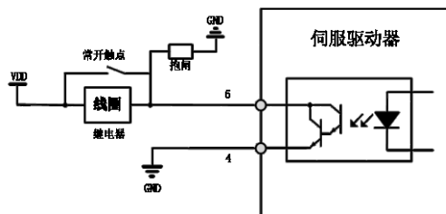
图 3-3 抱闸接线示意图
