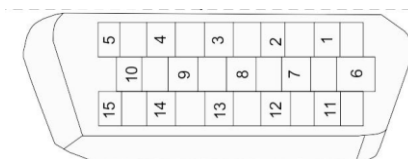
图 3-2 CN3 焊线端脚号图
