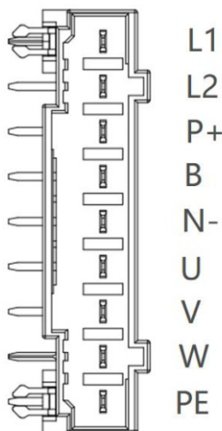
图 3-1 端子排分布图
