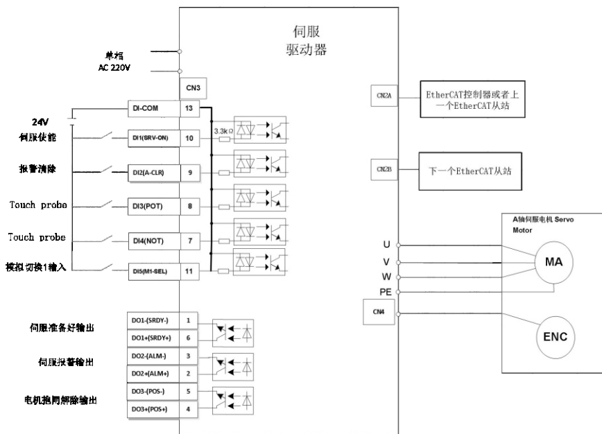
图 3-5 TSVC-EA 系列控制接线连接图
