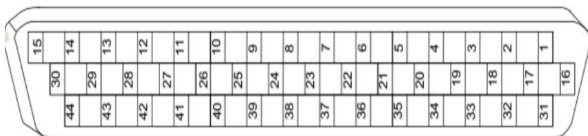
图 3-2 CN3 焊线端脚号图
