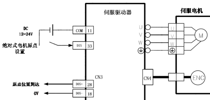
图 7-5 绝对式电机回零接线示意图
