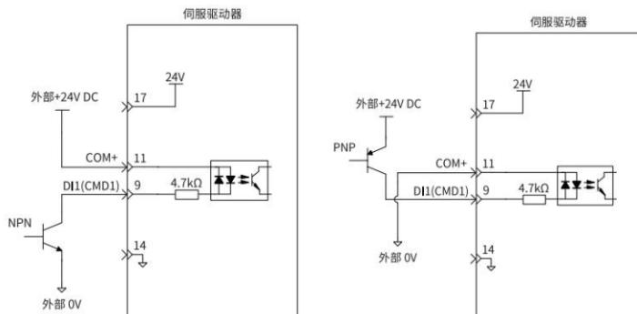
图 3-8 使用外部部电源
