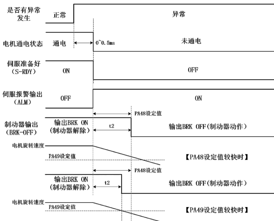
图 5-12 报警时序
