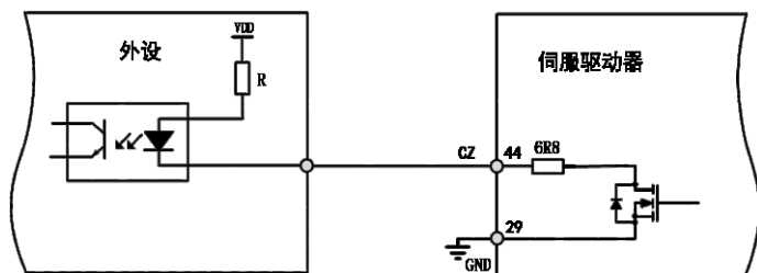
图 3-10 编码器 Z 信号集电极开路输出
