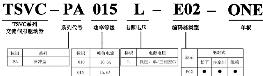
图 2-2 TSVC 脉冲系列交流伺服驱动器命名规则
