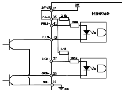
图 3-4 内部电源集电路接线方式
